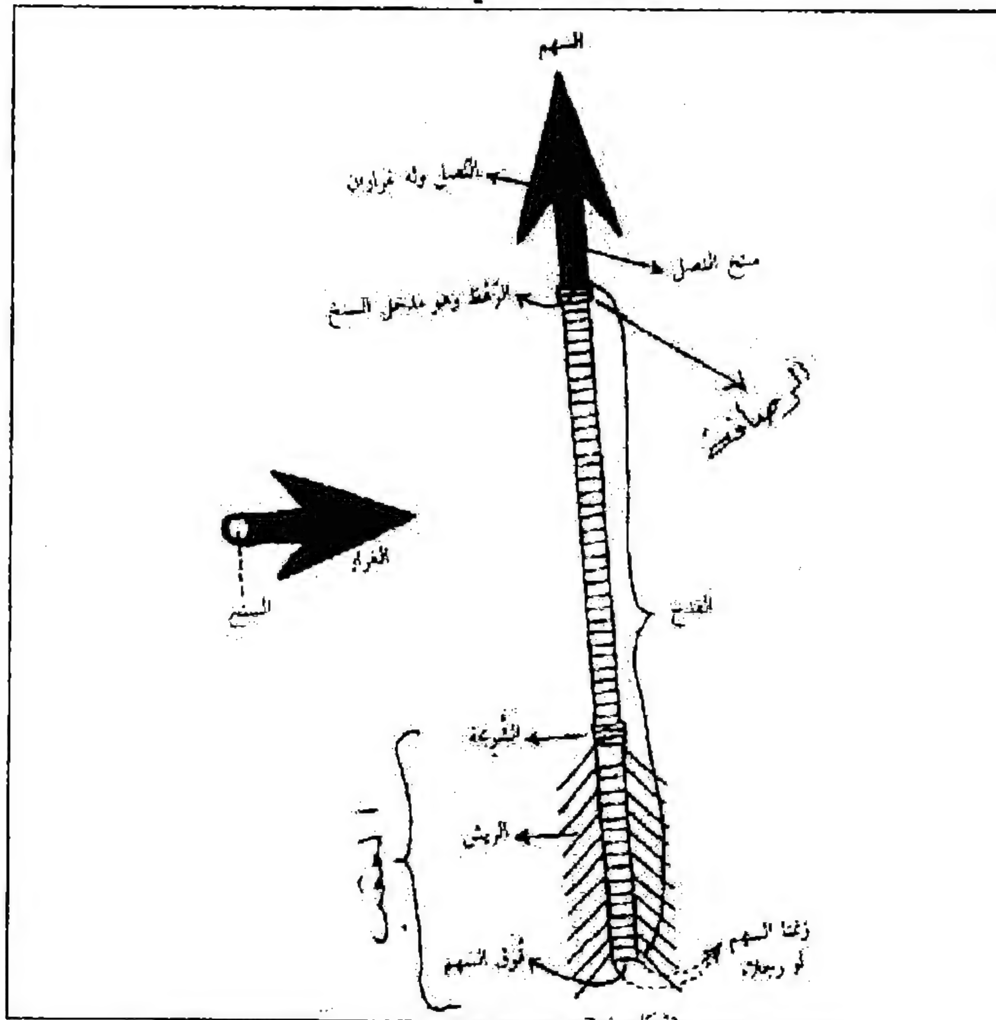
الشكل رقم (٤) المحتوى (أجزاء السهم)
